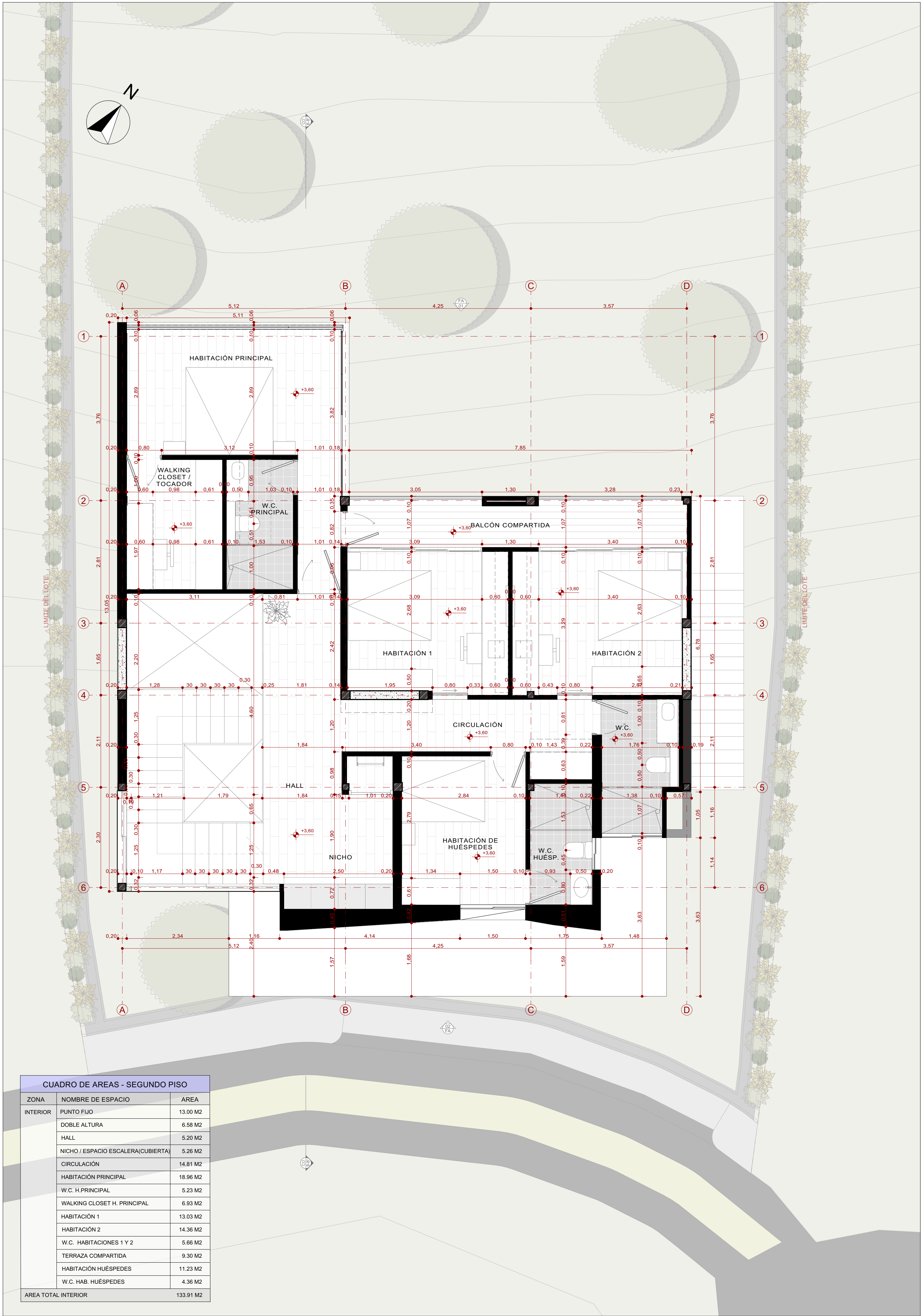
Plano de Segundo Piso:
